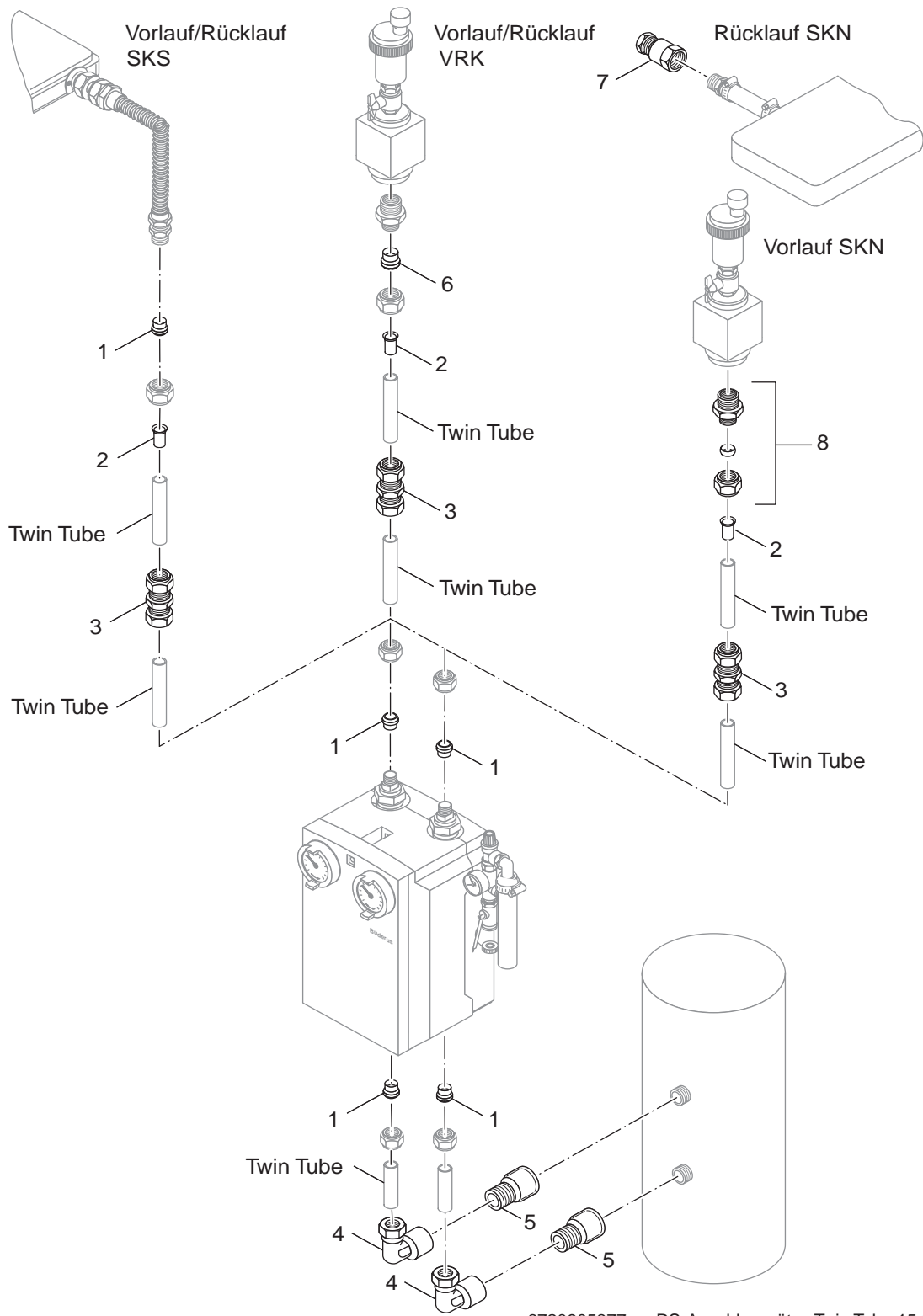
6720905877.aa.RS-Anschlusssätze Twin Tube 15 SKS/SKN/VRK
