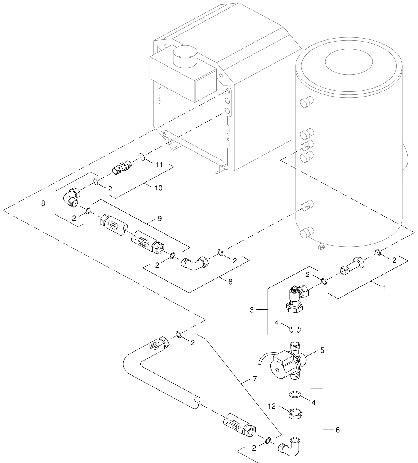
99900122.aa.RS-Kessel-Speicherverrohrung G134X SU
