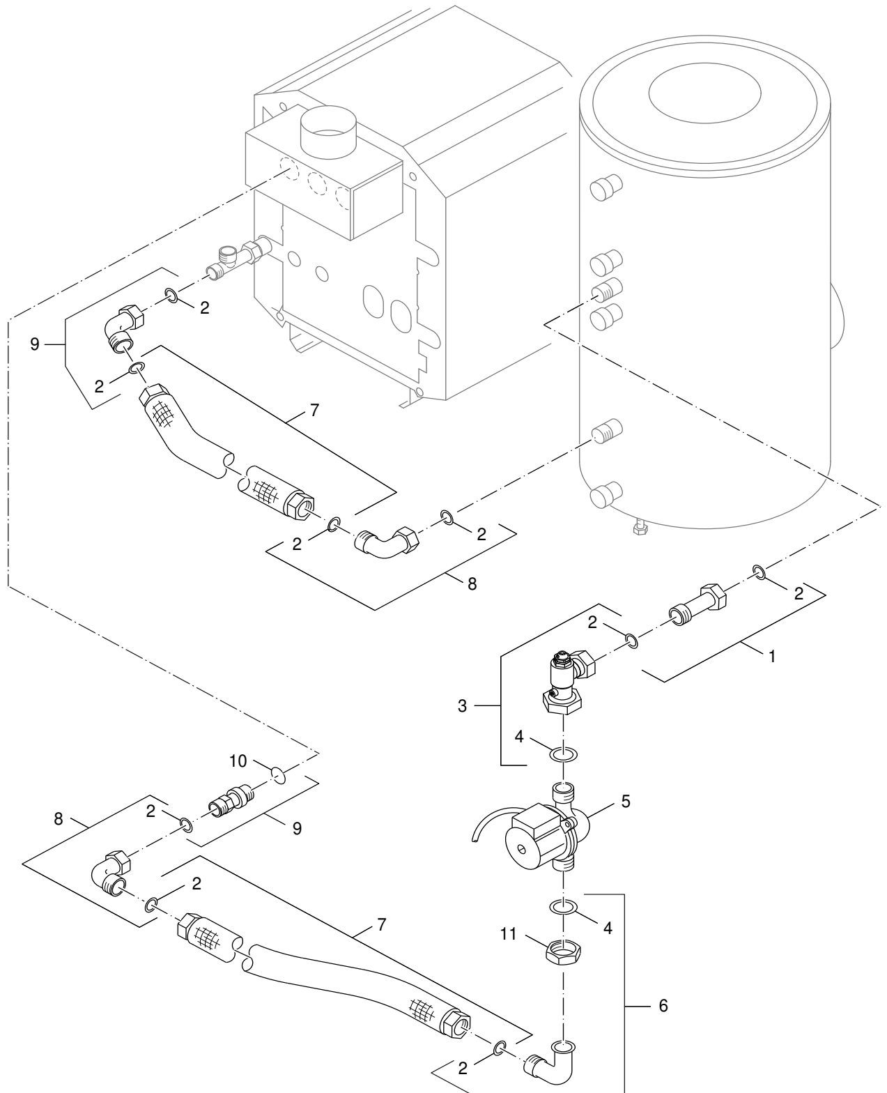
99900123.aa.RS-Kessel-Speicherverrohrung G124X/124 SU
