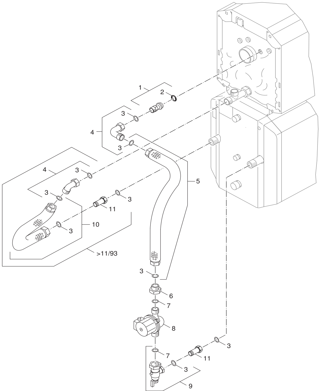
99909319.aa.RS-Rohrgruppe G1 15/G(B)125 LT135/160/200-LT135/1-160/1-200/1
